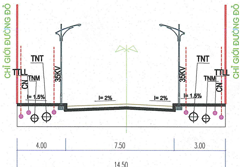
MẶT CẮT 3 - 3
