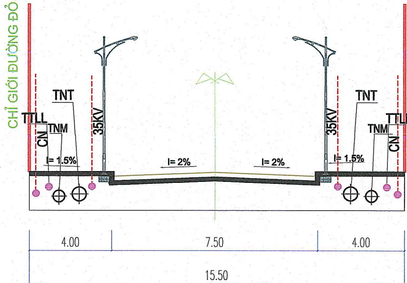
MẶT CẮT 2 - 2
