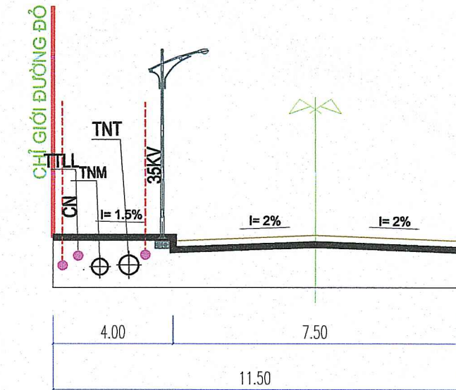
MẶT CẮT 1 - 1
