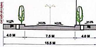
MẶT CẮT 1 - 1 (ĐƯỜNG QUY HOẠCH 1 VÀ ĐƯỜNG HIỆN CÓ)
